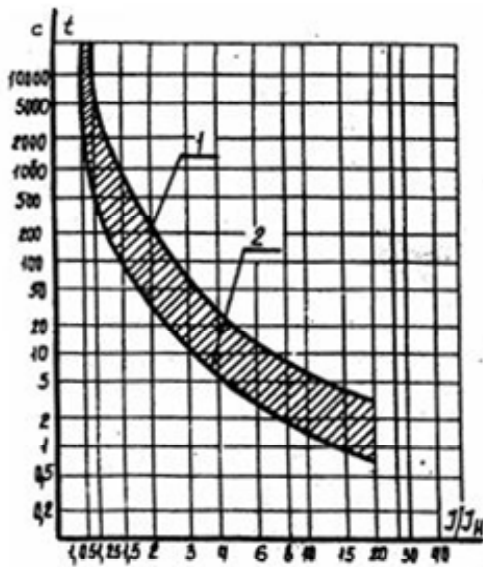
1 - верхний предел калибровки. 2 - нижний предел калибровки.
