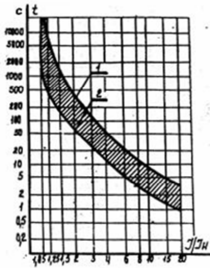
A3700 на ток 25,32,100 и 160А. 1 - верхний предел калибровки. 2 - нижний предел калибровки.
