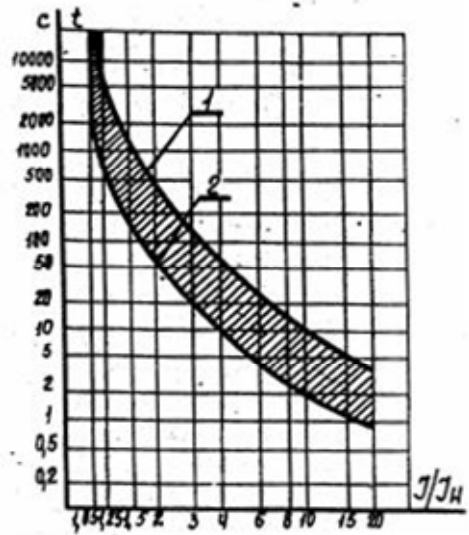
A3700 на ток 160,200,250А. 1 - верхний предел калибровки. 2 - нижний предел калибровки.
