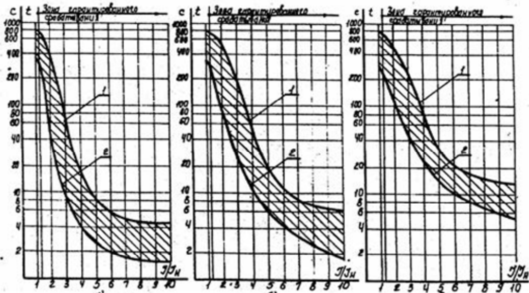
Защитные характеристики полупроводниковых расцепителей переменного тока.
