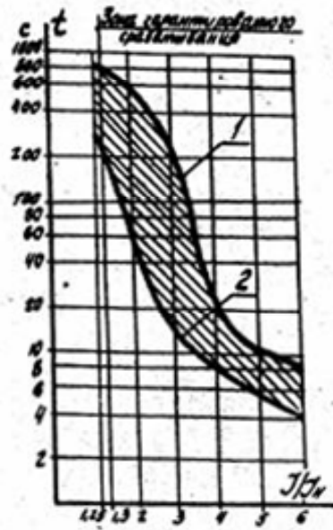
Защитные характеристики полупроводниковых расцепителей постоянного тока.
