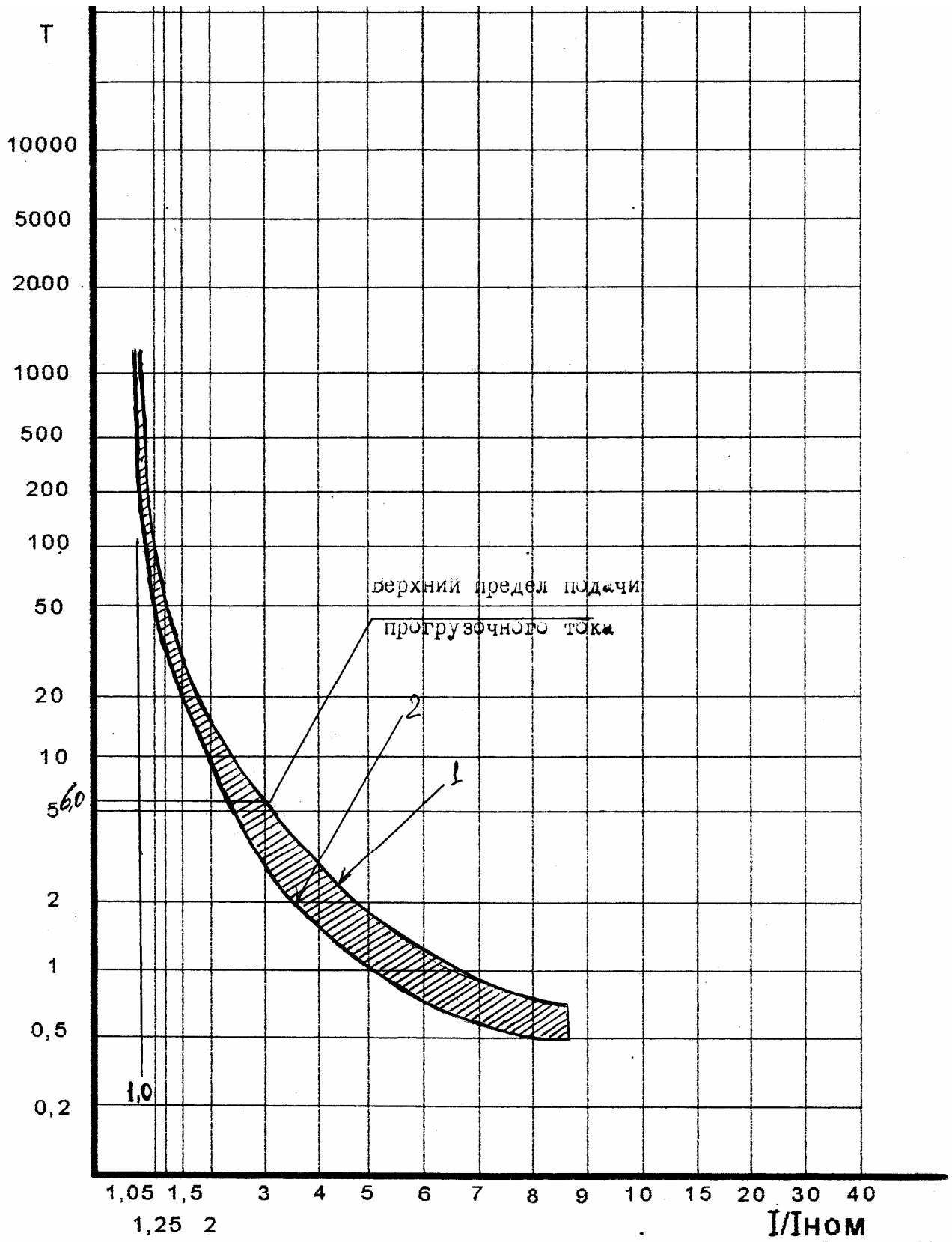
Защитные характеристики автоматического выключателя АРМ - 50
