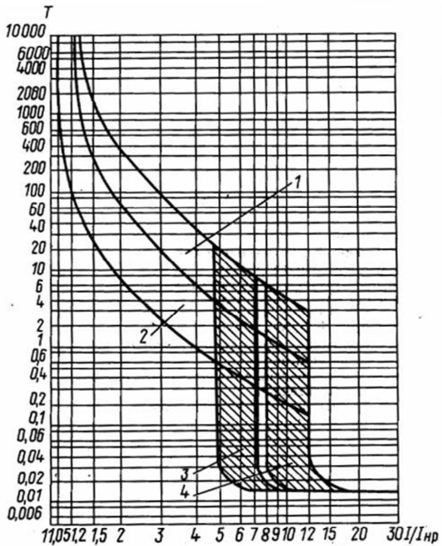
Времятоковая характеристика выключателей серии ВА51-39 и ВА52-39
