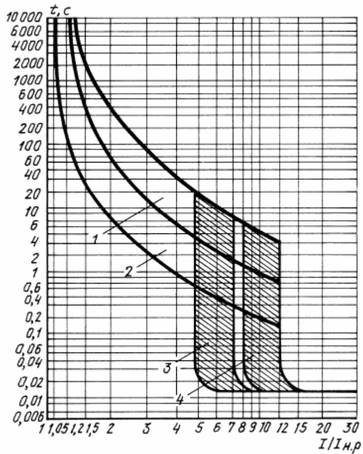
Время-токовые характеристики выключателей BA52-37:
