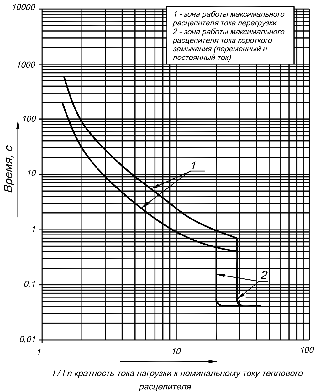
Время-токовые характеристики с холодного состояния выключателя на 16А
