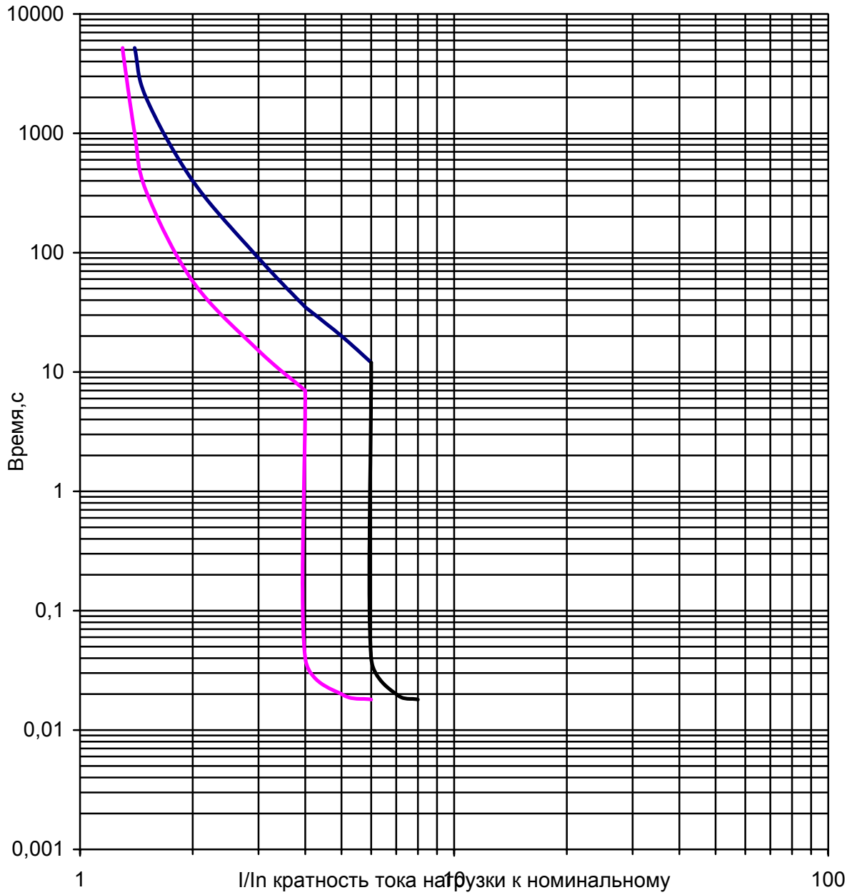
Характеристики с холодного состояния. Уставка электромагнитного
