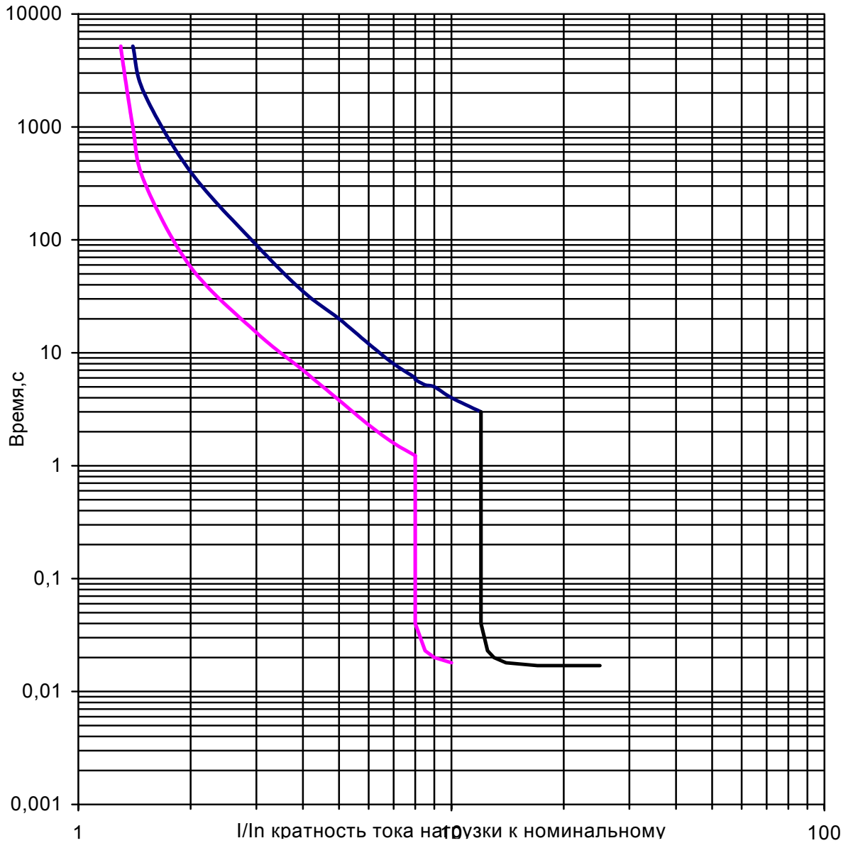
Характеристики с холодного состояния. Уставка электромагнитного
