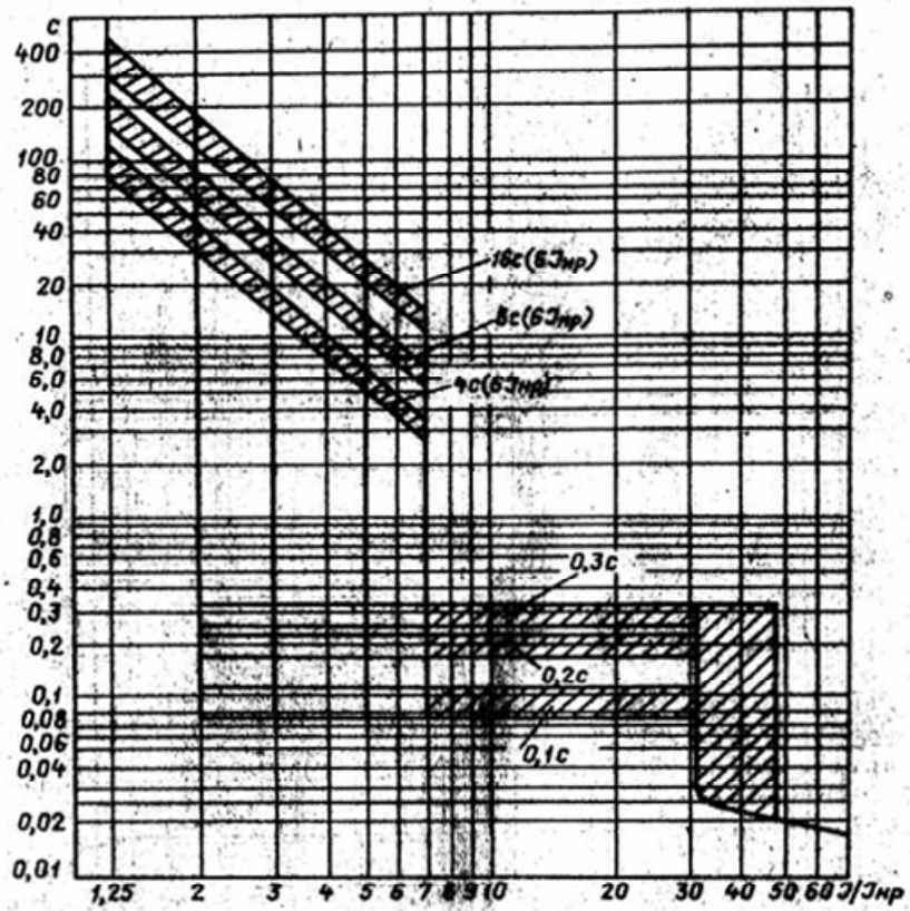
Времятоковая характеристика выключателей серии BA55-41 на 630А
