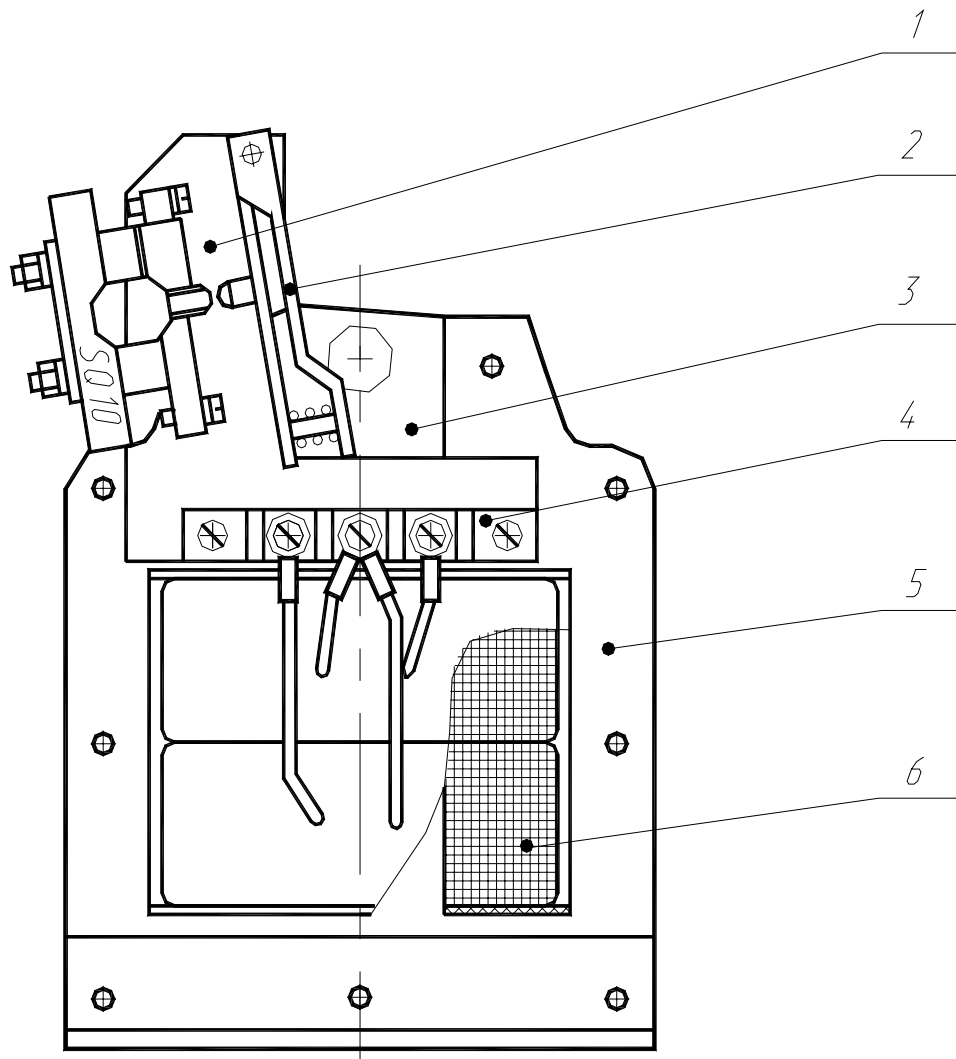
Электромагнит включения Рисунок 7
