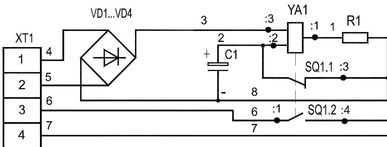
Рисунок 5. Схема электрическая принципиальная расцепителя минимального напряжения.
