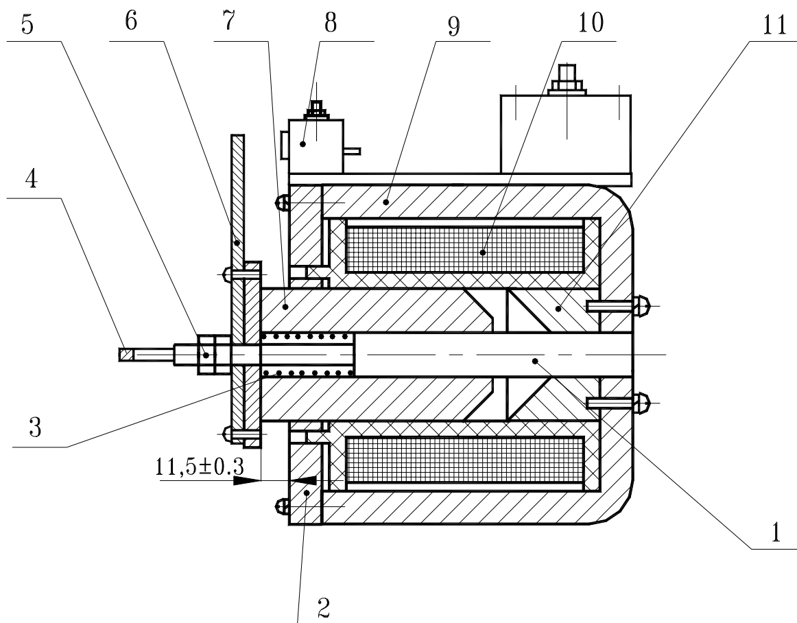
Расцепитель с питанием от независимого источника Рисунок 6
