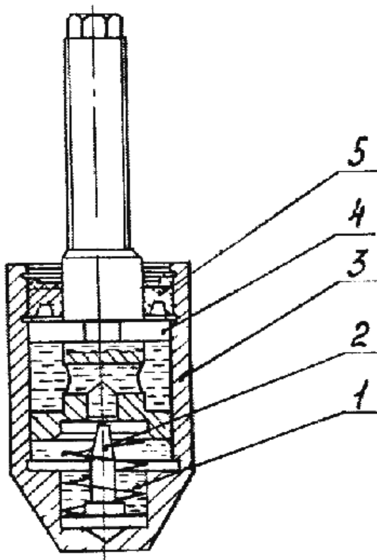
Демпфер Рисунок 9
