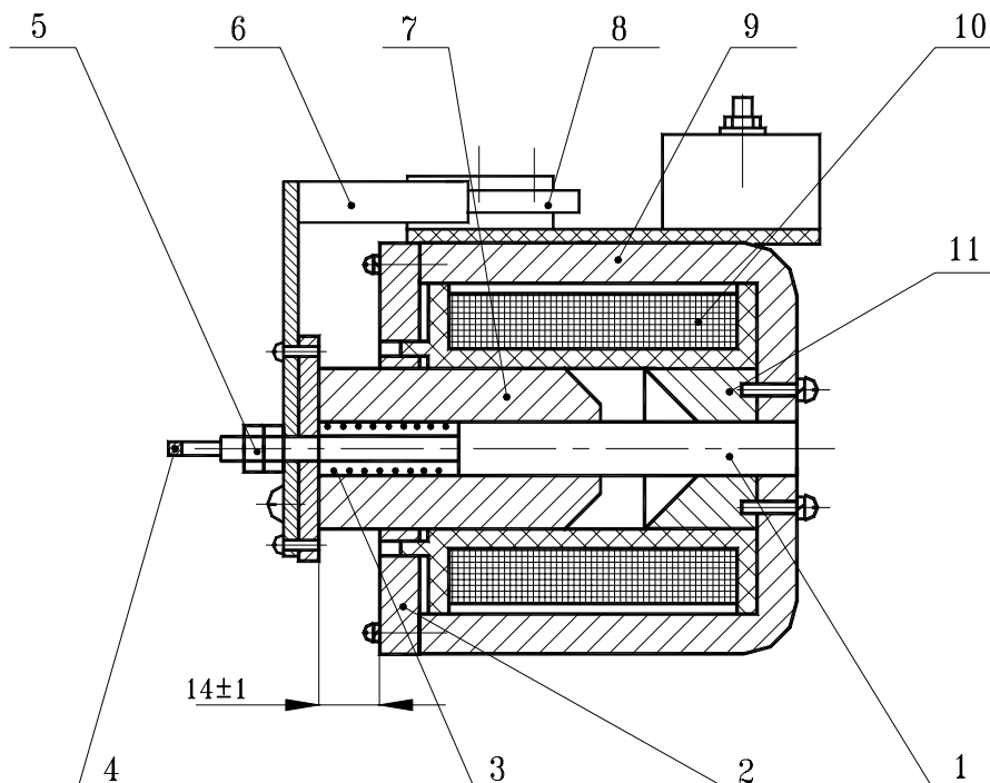
Расцепитель максимального тока Рисунок 2
