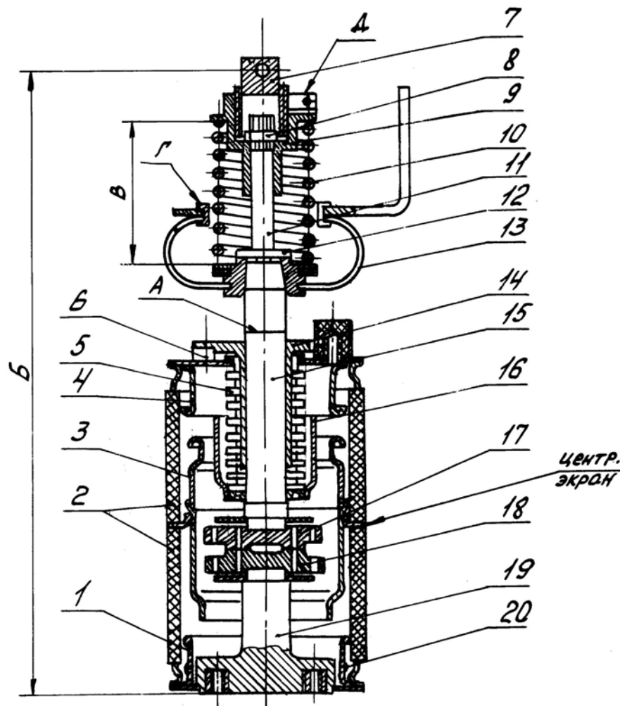
Дугогасительный блок Рисунок 1
